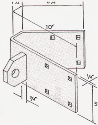
45° Corner Hinge Plate 1 Tab (Male) 6H412
