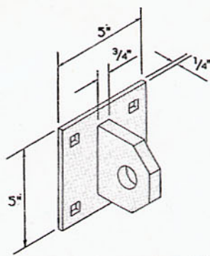
T-Hinge Plate 1 Tab (Male) 6H404
