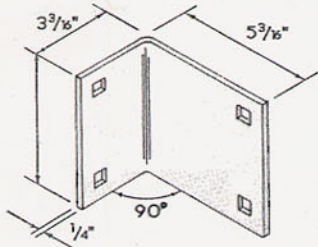
90° Stiffener Plate 6H414
